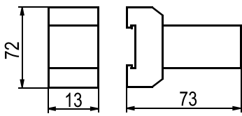
Рисунок 3. Реле с розеткой типа 2
