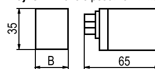
Рисунок 2. Реле с розеткой типа 1
