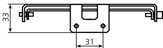
Скоба реле РЭО-401
