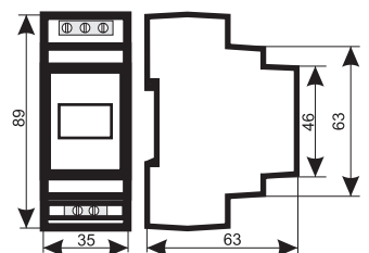
Габаритные размеры
