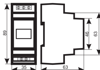
Габаритные размеры
